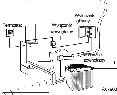
Rys. 1 – Wyłączniki elektryczne
